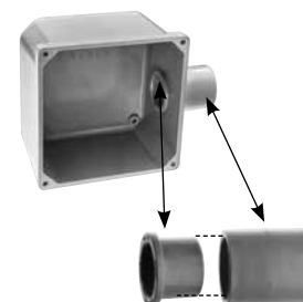
Adaptateur pour boite de jonction Manchon standard en PVC
