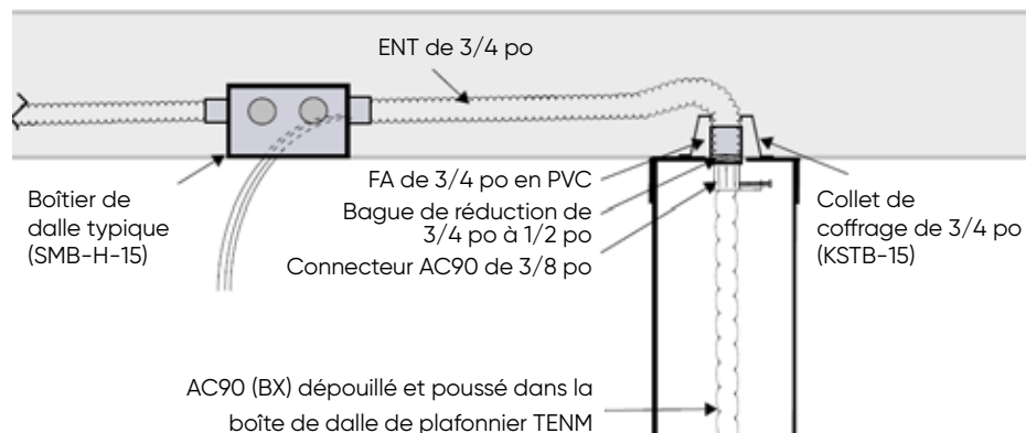
Dalle typique
