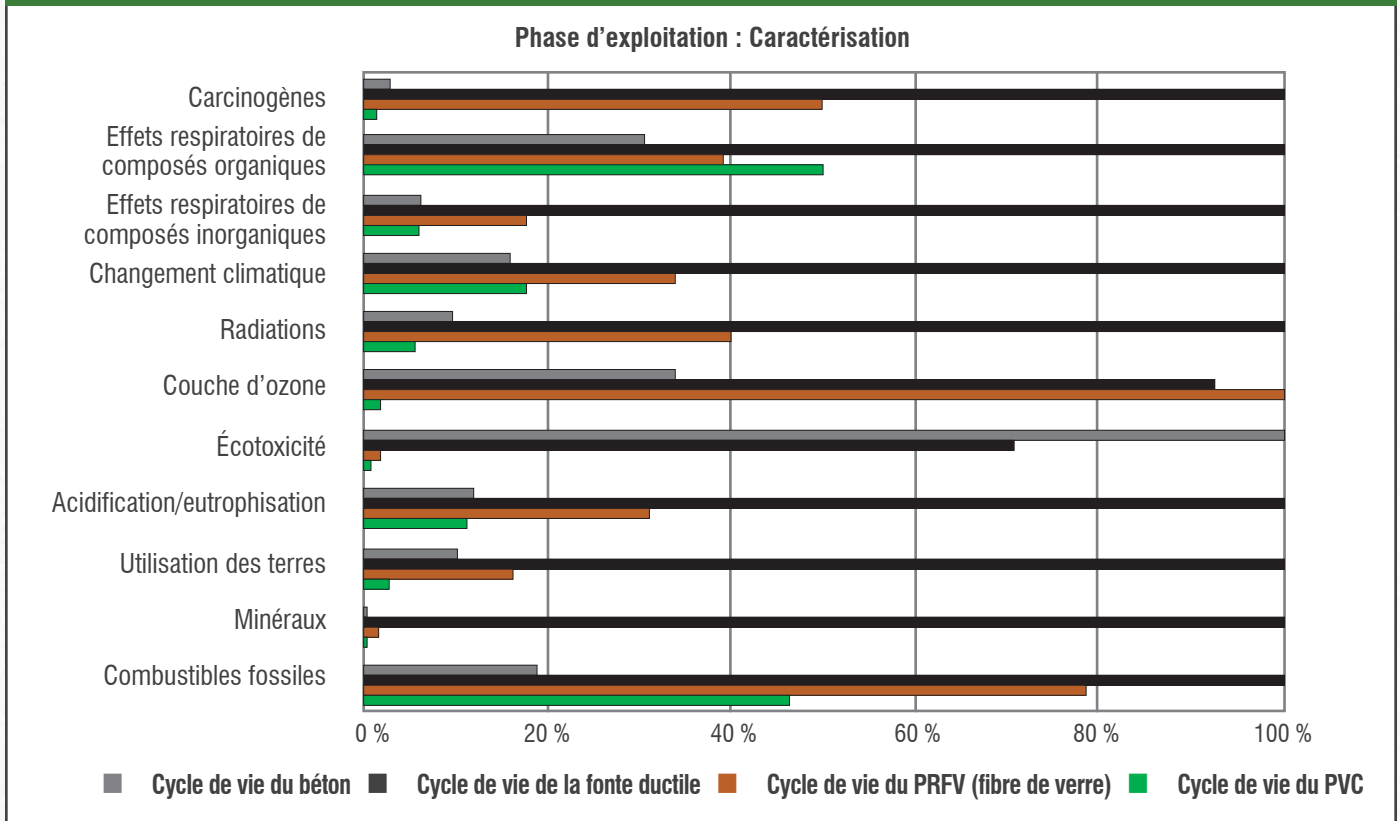
FIGURE A.27 : GRAPHIQUE DE CARACTÉRISATION DE LA COMPARAISON DU CYCLE DE VIE POUR TOUS LES MATÉRIEAUX DE TUYAUX
