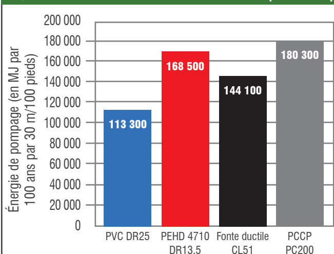
FIGURE A.18 : ÉNERGIE DE POMPAGE SUR 100 ANS DE TUYAUX ÉQUIVALENTS AUX TUYAUX PVC DR25 DE 600 MM (24 POUÇES)
