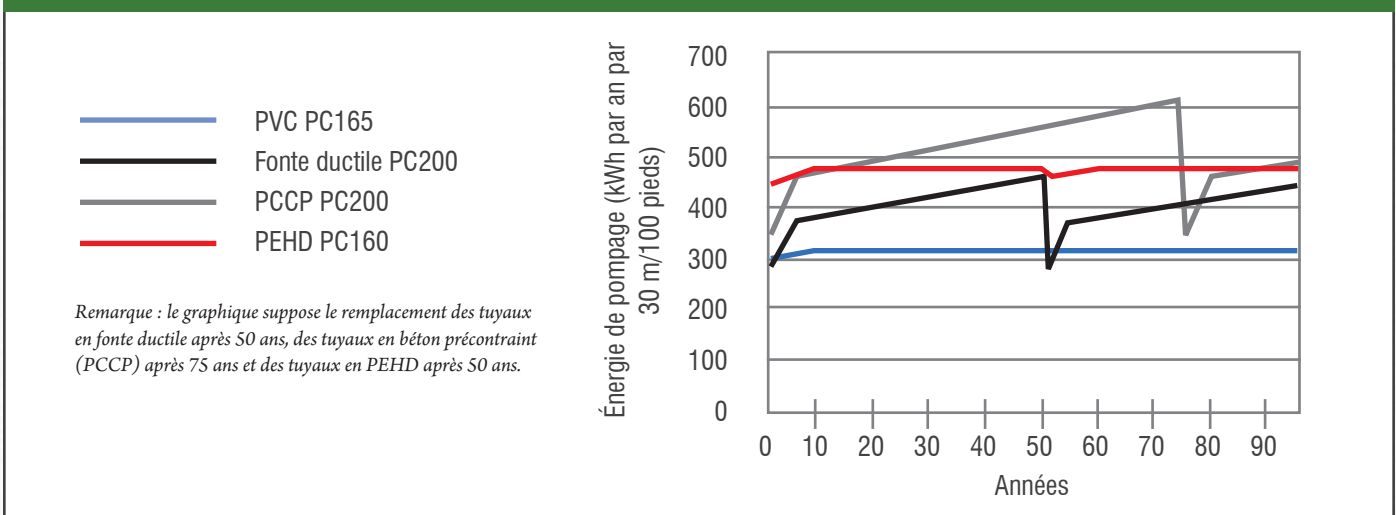
FIGURE 8.4 : COMPARAISON DES CONSOMMATIONS ÉNERGÉTIQUES ANNUELLES DE POMPAGE POUR DES TUYAUX DE 600 MM (24 POUÇES)
