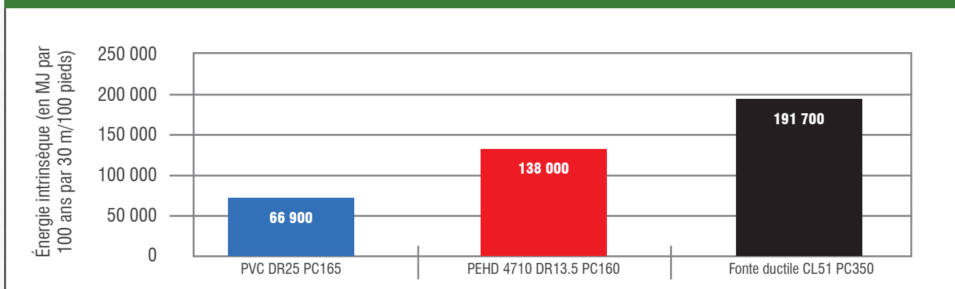
FIGURE A.6 : TUYAUX EN PVC ÉQUIVALENTS DR25 DE 200 MM (8 POUCES) : ÉNERGIE INTRINSÈQUE TOTALE SUR 100 ANS
