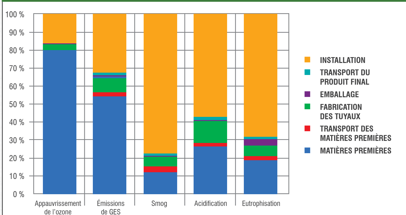
FIGURE 4.4 : IMPACTS ENVIRONNEMENTAUX DES TUYAUX D'ÉGOUTS SANITAIRES DE 200 MM (8 POUÇES) EN PVC À PARI PLEINE PS46 SDR35 ASTM D3034 (EN UTILISANT LA MÉTHODOLOGIE DE CALCUL DES IMPACTS TRACI)
