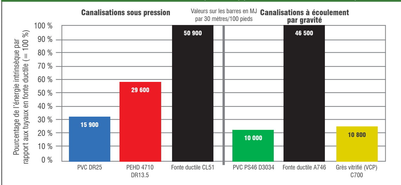
FIGURE A.14 : COMPARAISON DES VALEURS DE L'ÉNERGIE INTRINSÈQUE DE LA CRÉATION À LA SORTIE D'USINE POUR DES TUYAUX EN PVC ÉQUIVALENTS DR25 DE 200 MM (8 POUCHES) (EN MJ PAR 30 MÈTRES/100 PIEDS)
