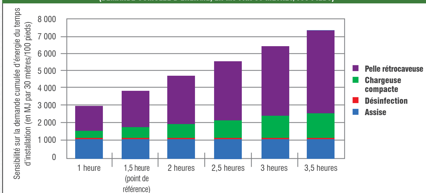
FIGURE 6.2: ANALYSE DE SENSIBILITÉ DES TEMPS D'INSTALLATION DE TUYAUX SOUS PRESSION DE 200MM (8 POUÇES) DE DIAMÈTRE DE 30 M (100 PIEDS) DE LONG (DEMANDE CUMULÉE D'ÉNERGIE, EN MJ PAR 30 MÈTRES/100 PIEDS)
