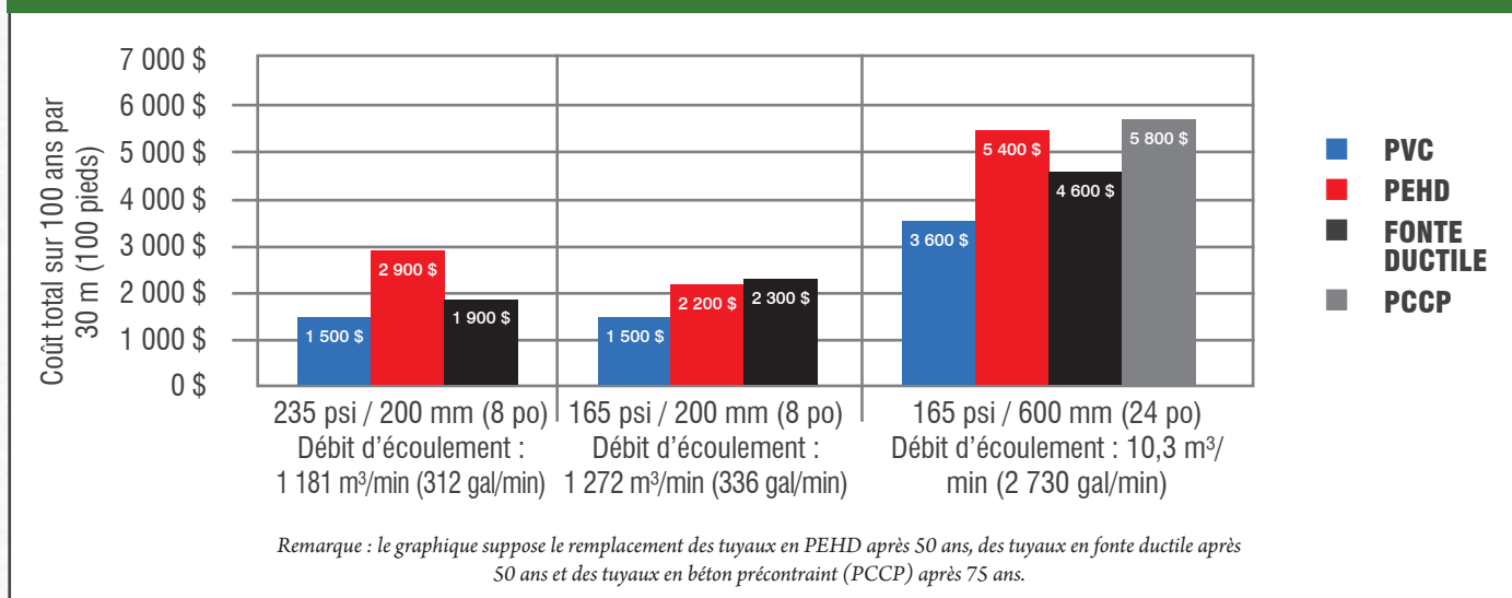
FIGURE A.4 : COÛT ÉNERGÉTIQUE DE POMPAGE SUR 100 ANS, POUR 30 MÈTRES (100 PIEDS) DE TUYAU
