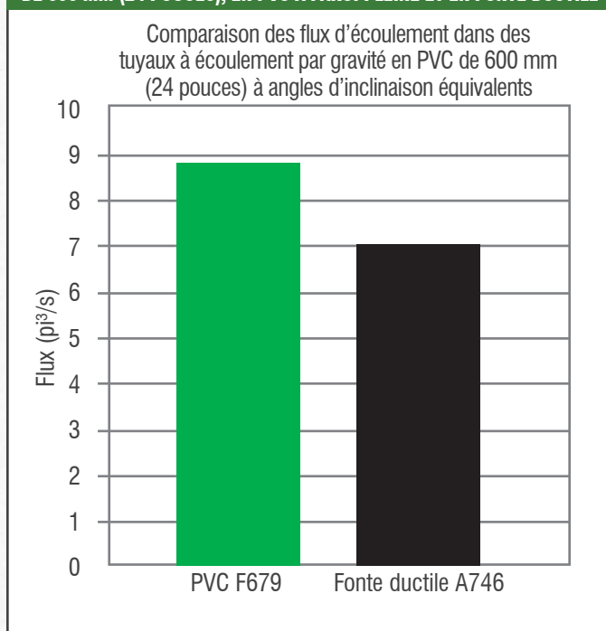
FIGURE 9.3 : COMPARAISON DES FLUX D'ÉCOULEMENT DANS DES TUYAUX DE 600 MM (24 POUÇES), EN PVC À PAROI PLEINE ET EN FONTE DUCTILE
