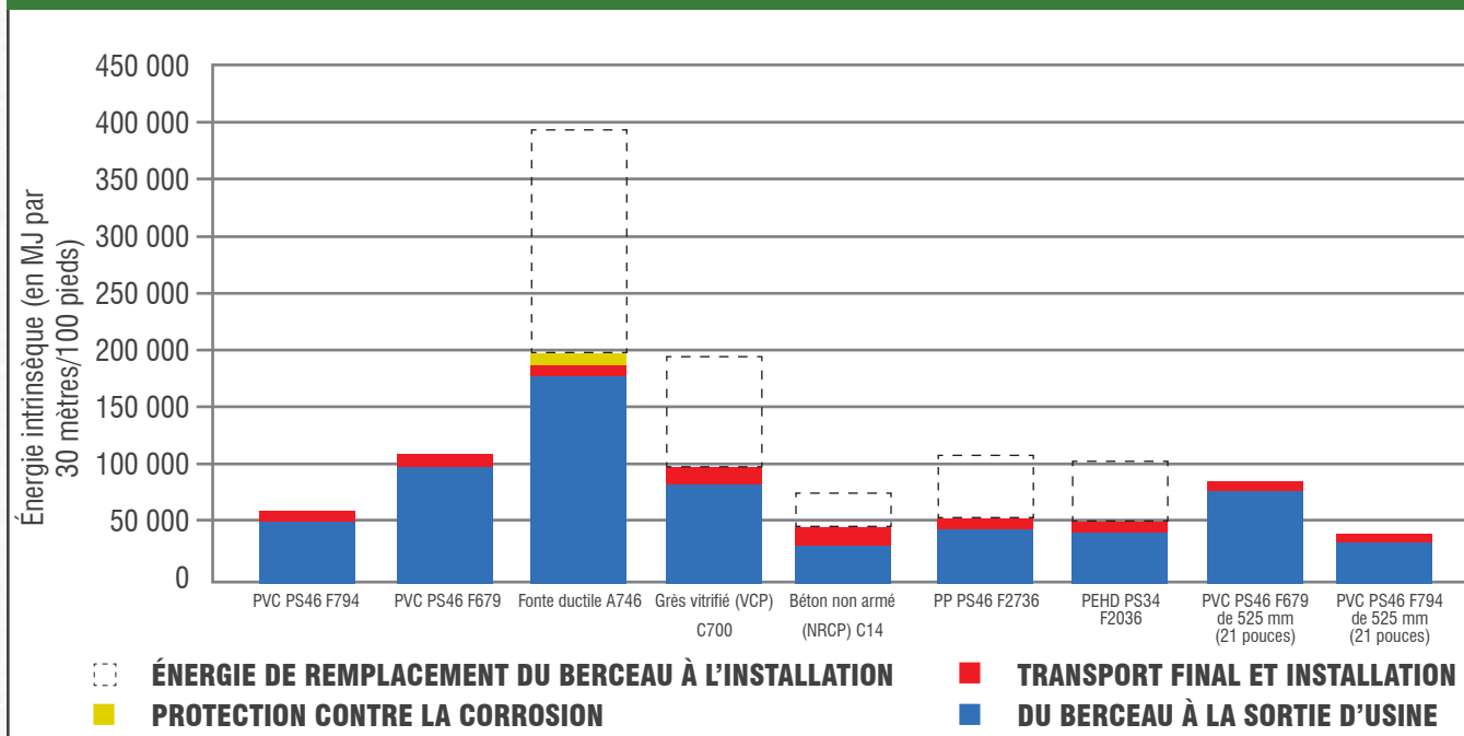
FIGURE 12.10: ÉNERGIE INTRINSÈQUE TOTALE SUR 100 ANS DE TUYAUX EN PVC ÉQUIVALENTS PS46 À PAROI PLEINE OU PAROI NERVURÉE DE 600 MM (24 POUÇES)
