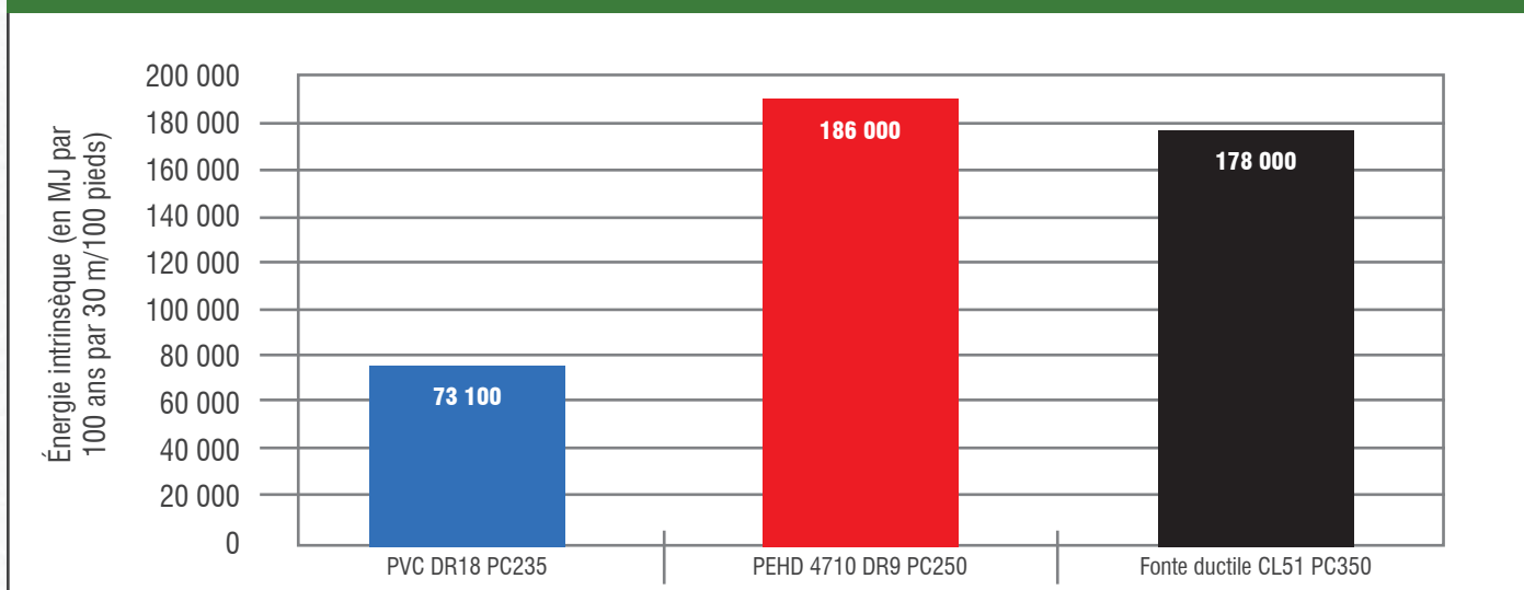
FIGURE A.5 : TUYAUX EN PVC ÉQUIVALENTS DR18 DE 200 MM (8 POUCES) : ÉNERGIE INTRINSÈQUE TOTALE SUR 100 ANS
