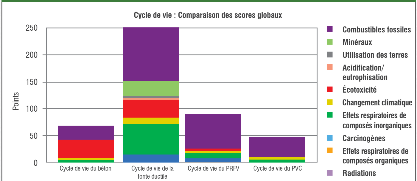
FIGURE A.28 : GRAPHIQUE DES SCORES GLOBAUX DE LA COMPARAISON DU CYCLE DE VIE POUR LES DIVERS MATÉRIEAUX DE TUYAUX
